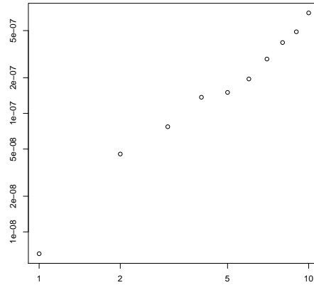
(D) Empirical 6^{\text{th}} moment \hat{m}_6(h) .
