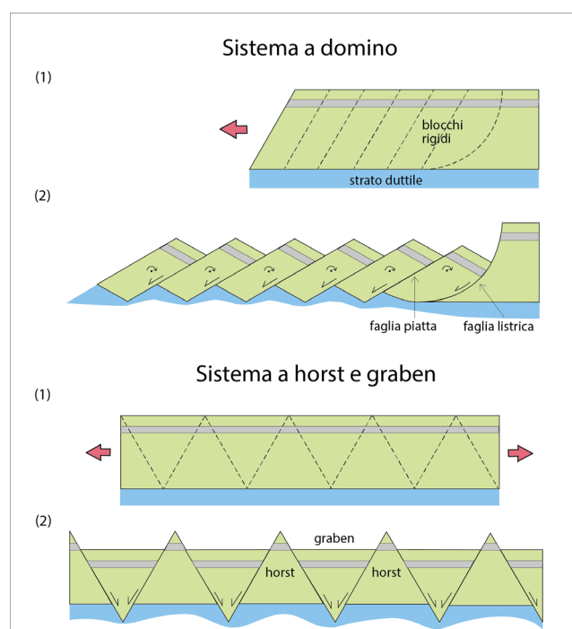
Fig. 2 - Modelli dell'estensione crostale tramite sviluppo di sistema a domino (faglie sintetiche) e sistema a horst e graben (faglie antitetiche).
