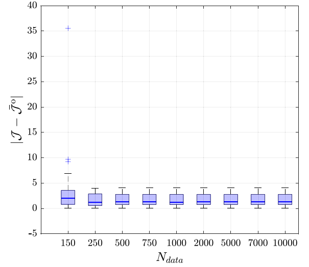
(a) |\mathcal{J} - \bar{\mathcal{J}}^o| vs N_{data}
