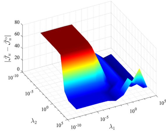
(b) |\mathcal{J}_u - \bar{\mathcal{J}}_u^o| vs \lambda_1 and \lambda_2
