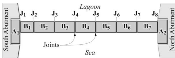
Figure 27. S.Nicolò barrier: plan view.
