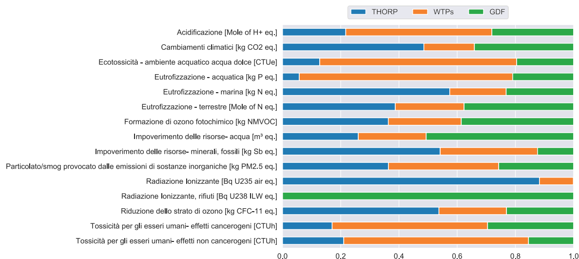
Figura 5 – Analisi hot-spot
