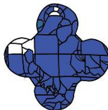
Rilievo del fenomeno di esfoliazione delle grisaglie
