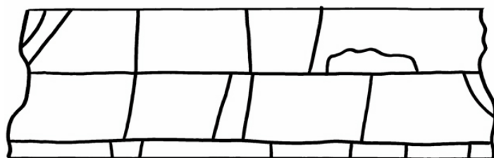
Rilievo del tracciato della tramatura plumbea
