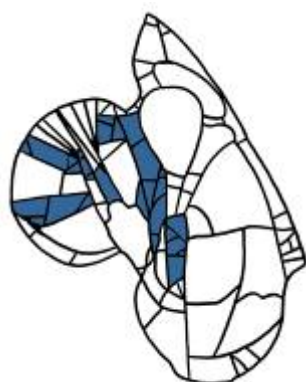
Rilievo del fenomeno di esfoliazione delle grisaglie
