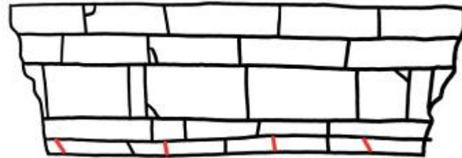
Rilievo di: fratture ——— suture ———
