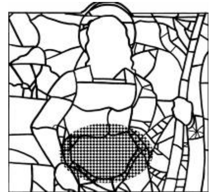
Rilievo delle spanciature verso l'interno ■■■■ verso l'esterno ■■■■
