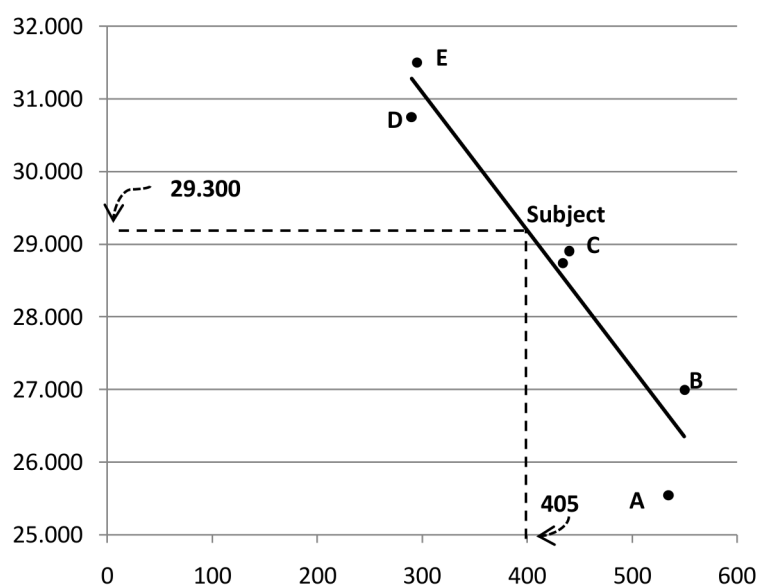
Grafico 2.2 - Price-quality regression tratta da Ratcliff (1972) pag. 160.
