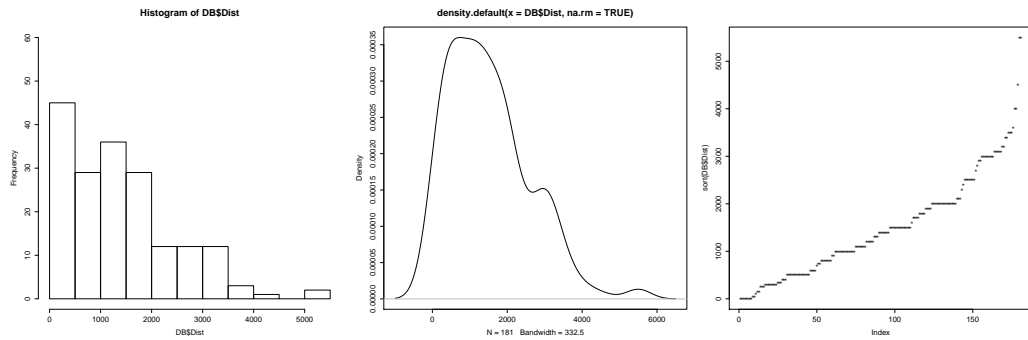
Grafico 3.2: Istogramma e grafici di distribuzione della variabile Dist
