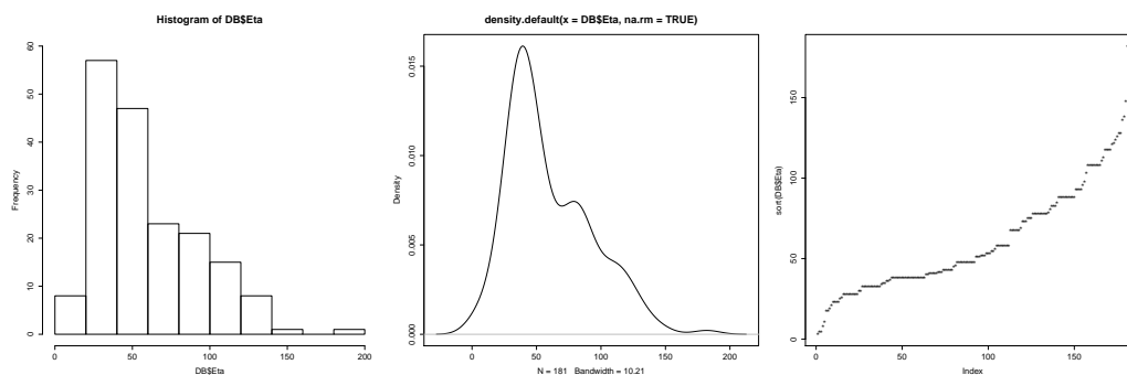
Grafico 3.4: Istogramma e grafici di distribuzione della variabile Eta
