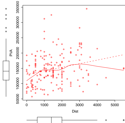
Grafico 3.3: Distribuzione del prezzo rilevato (PVA) rispetto alla distanza (Dist)
