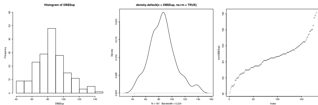
Grafico 3.6: Istogramma e grafici di distribuzione della variabile Sup
