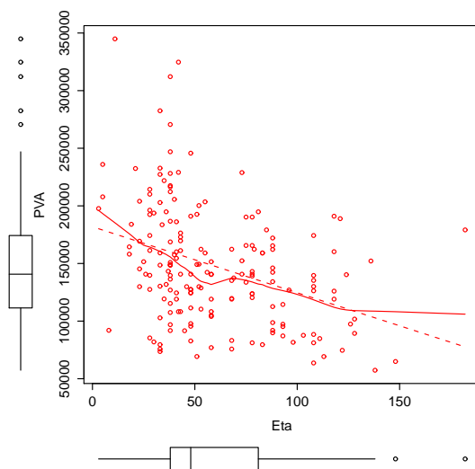
Grafico 3.5: Distribuzione del prezzo rilevato (PVA) rispetto alla distanza (Eta)
