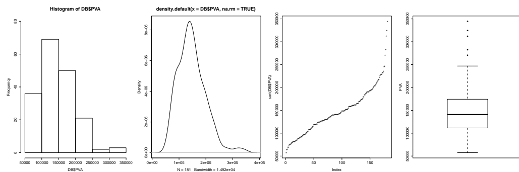
Grafico 3.1: Istogramma e grafici di distribuzione della variabile PVA
