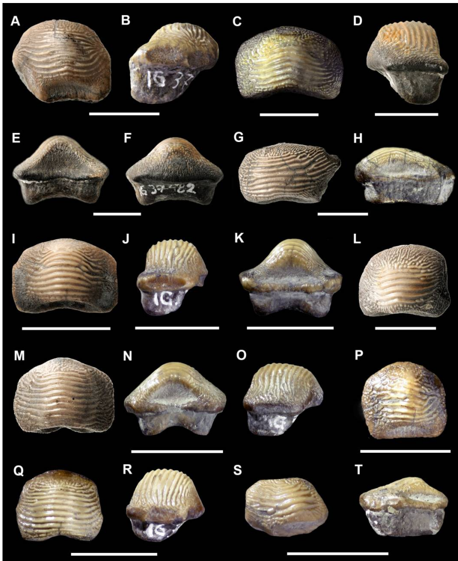
Fig. 6 - Ptychodus decurrens Agassiz, 1938; Bomba Quarry (Cinto Euganeo). MGCB IG37483, A) occlusal and B) lateral view; MGCB IG37482, C) occlusal, D) lateral, E) posterior view and F) anterior view; MGCB IG37481, G) occlusal and H) posterior view; MGCB IG37479, I) occlusal, J) lateral and K) posterior view; MGCB 446, L) occlusal view; MGCB IG37478, M) occlusal, N) posterior and O) lateral view; MGCB IG37477, P) occlusal view; MGCB IG37476, Q) occlusal and R) lateral view; MGCB IG37475, S) occlusal and T) posterior view. Scale bars equal 5 mm.
